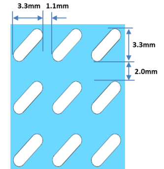
※ VENT Detailed Size (TOP)
