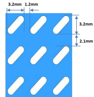
※ VENT Detailed Size (CENTER)
