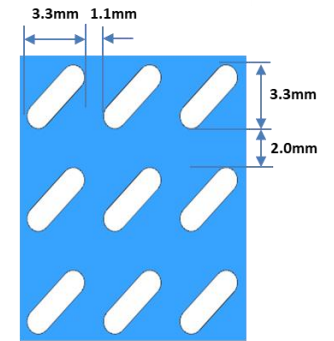
※ VENT Detailed Size (SIDE)
